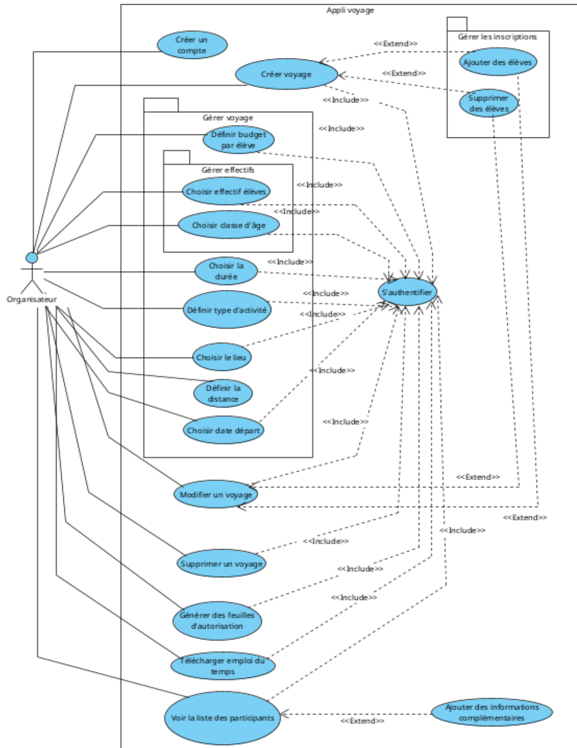
Figure 1. Diagramme de cas d'utilisation de l'application d'organisation de voyages scolaires
