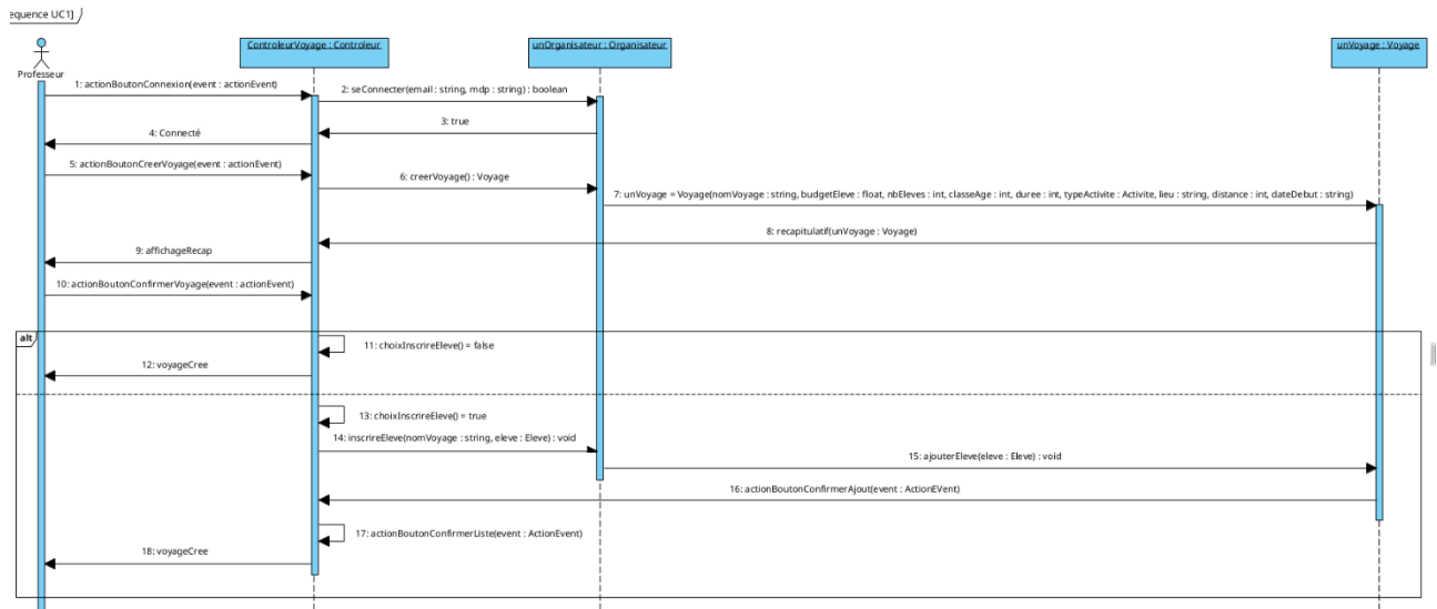
Figure 5. Diagramme de séquences détaillées du scénario nominal de UC1.
