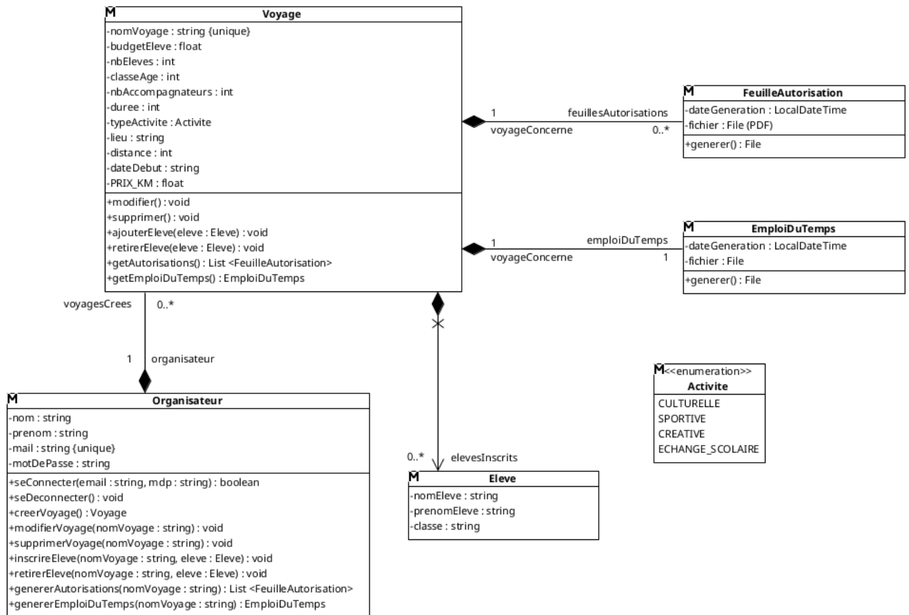
Figure 2. Diagramme de classe métier
