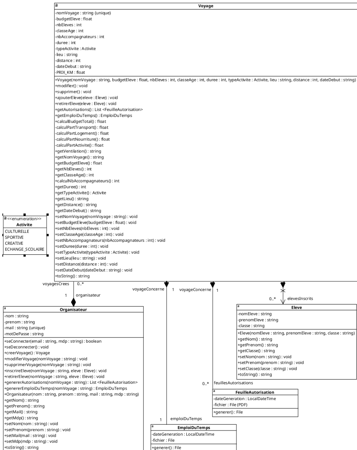
Figure 4. Diagramme de classe métier détaillé.
